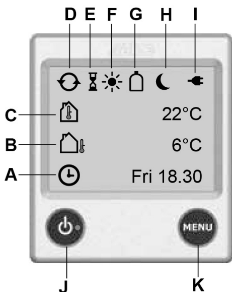
Afb. 137: Bedieningselementen
