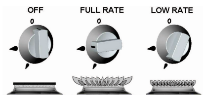
Afb. 182: Standen van de bedieningselementen: UIT, maximum, minimum
