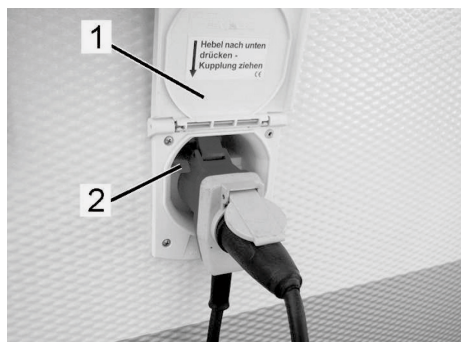
Afb. 101: Netaansluiting
