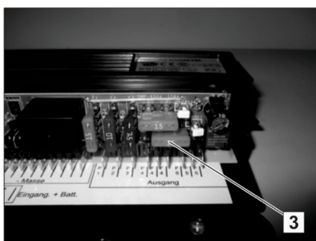
Afb. 64: Complete 12 V-voeding
