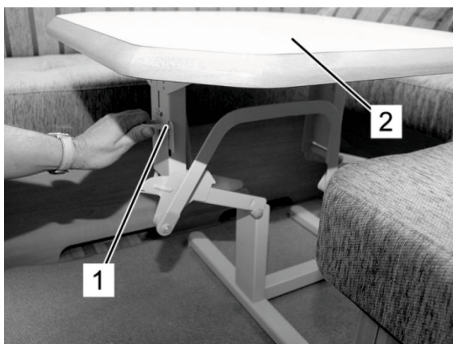
Afb. 153: tafel met heftafeldraagconstructie
