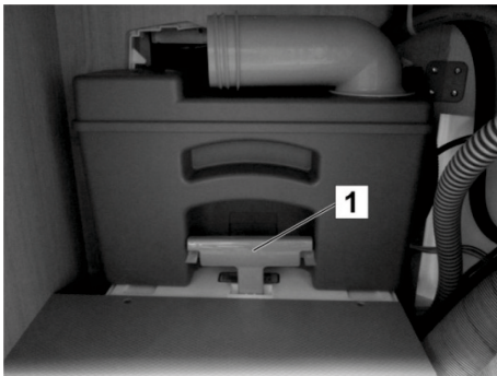
Afb. 175: Fecaliëntank in het afvalkanaal
