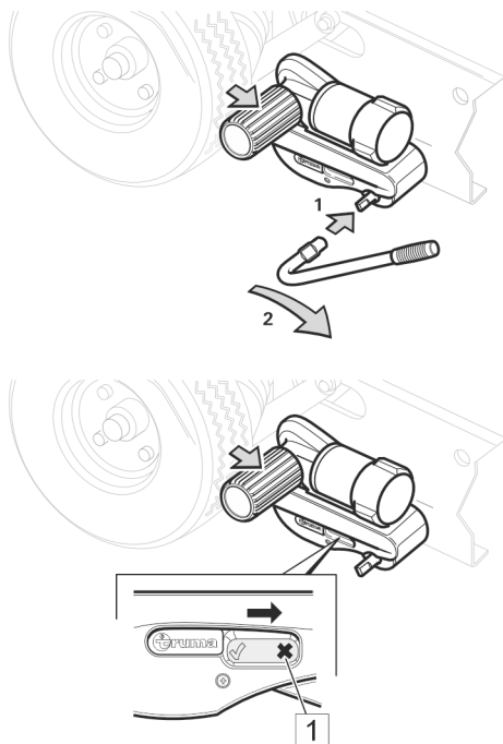
Afb. 13: Mover smart M uitzwenken
