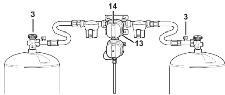
Afb. 116: Gasdrukregelset
