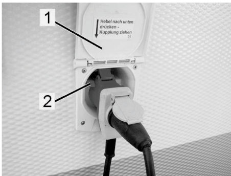
Afb. 61: Netaansluiting
