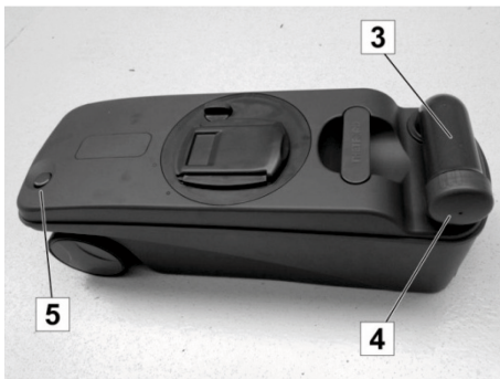
Afb. 173: Fecaliëntank legen
