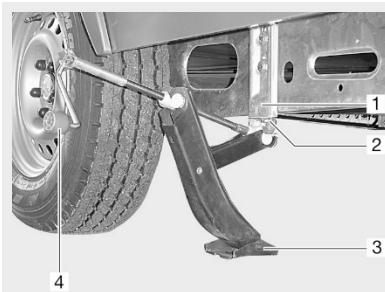
Afb. 195: Wagenkrik, AL-KO
