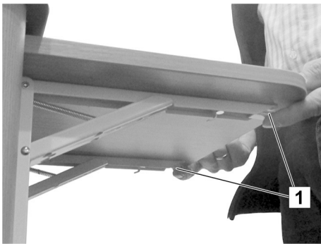
Afb. 188: Vergrendeling van de klapconsole losmaken
