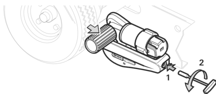
Afb. 14: Mover smart A handmatig uitzwenken
