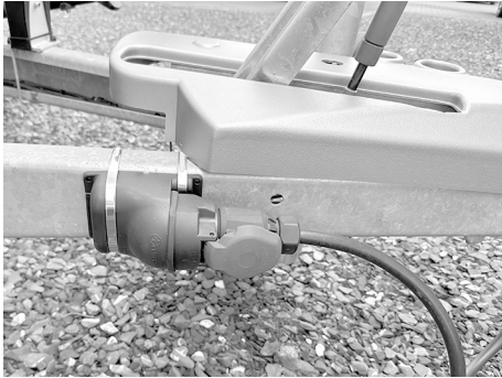
Afb. 11: stopcontact op de dissel
