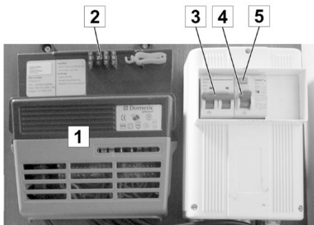
Afb. 62: Omvormer (netvoeding) (1) en zekeringautomaten
