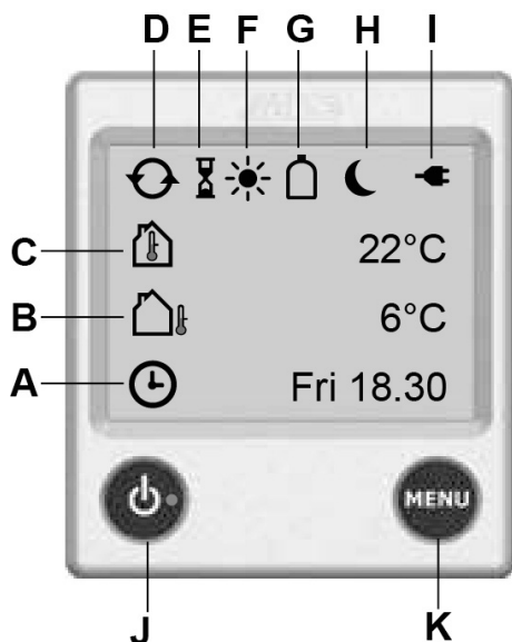
Afb. 86: Bedieningselementen
