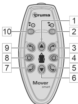
Afb. 10: Afstandsbediening Mover smart
